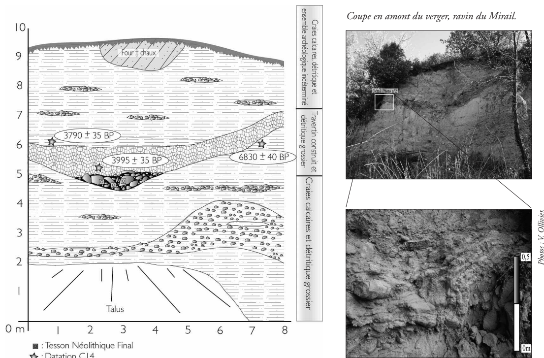
Fig. 4 : séquence travertineuse holocène en amont du Verger, ravin du Mirail, fluctuations hydro-sédimentaires et alternances de faciès travertineux.
