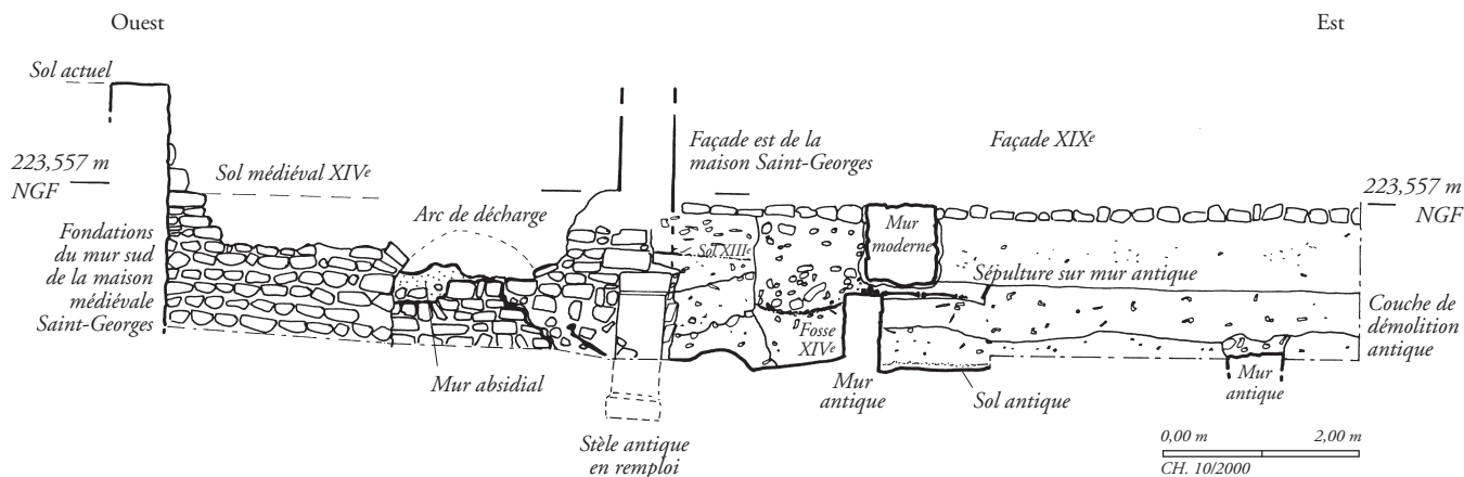
Fig.9 : site archéologique Saint-Georges : coupe ouest/est.
