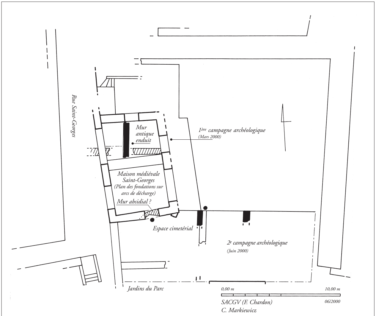
Fig.4 : site archéologique Saint-Georges : plan général du niveau des caves.
